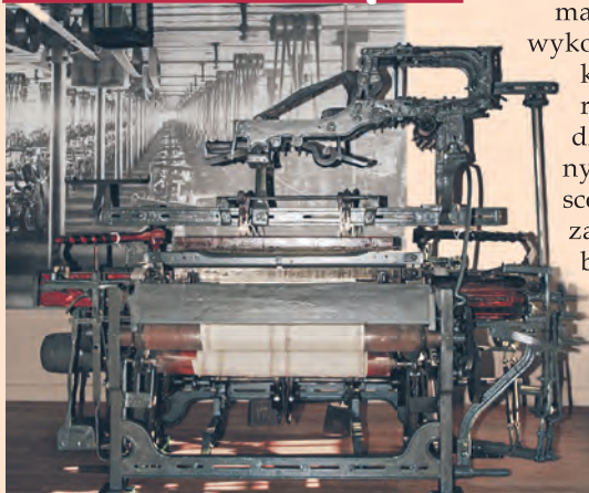
Krosno mechaniczne z maszyną nicielnicową
